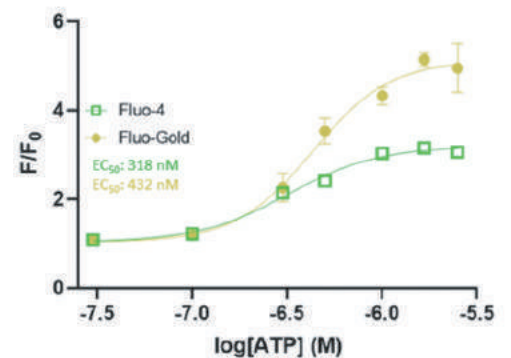
GPCR Assay
