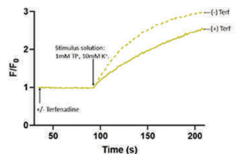
hERG ( K_v 11.1) Assay
